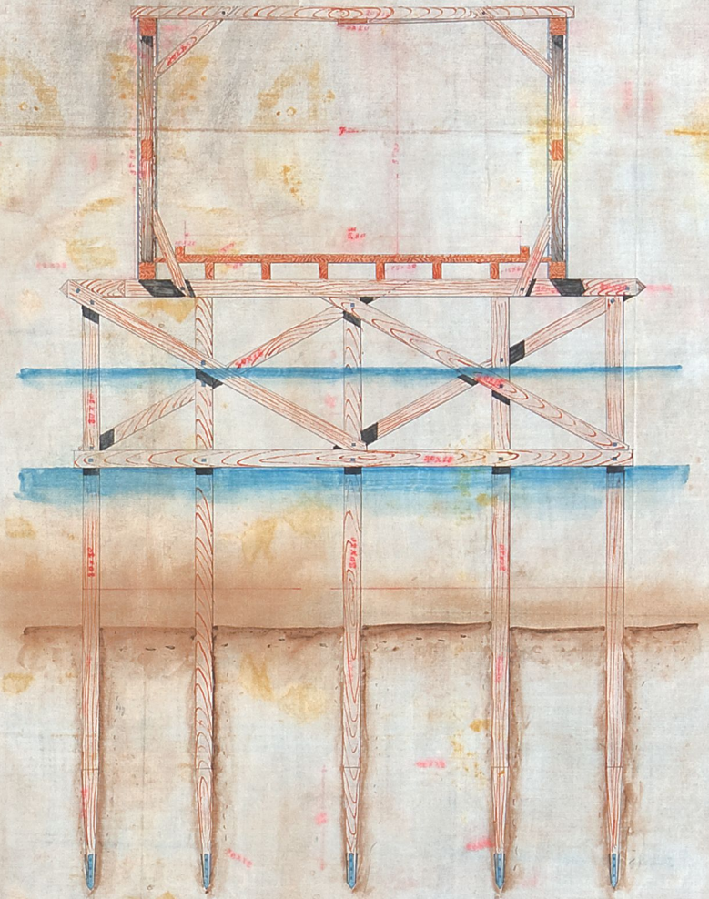
Corte Transversal
