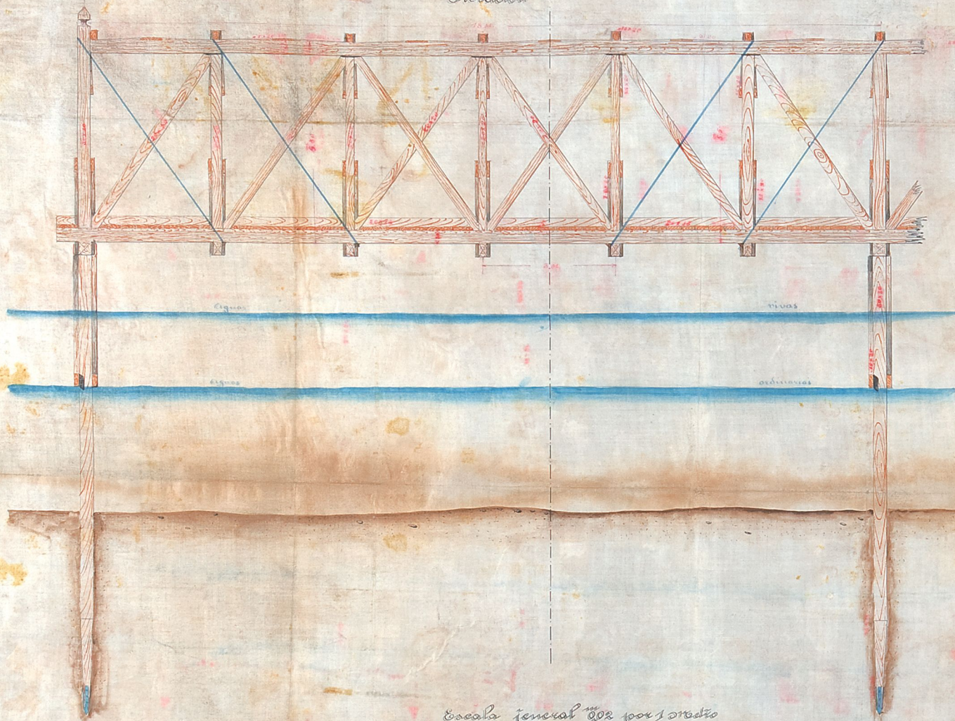
Elevación
