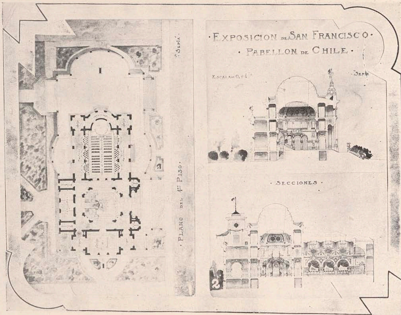
Corte y Plano del Proyecto Exposición de San Francisco «Pabellón Chile».
