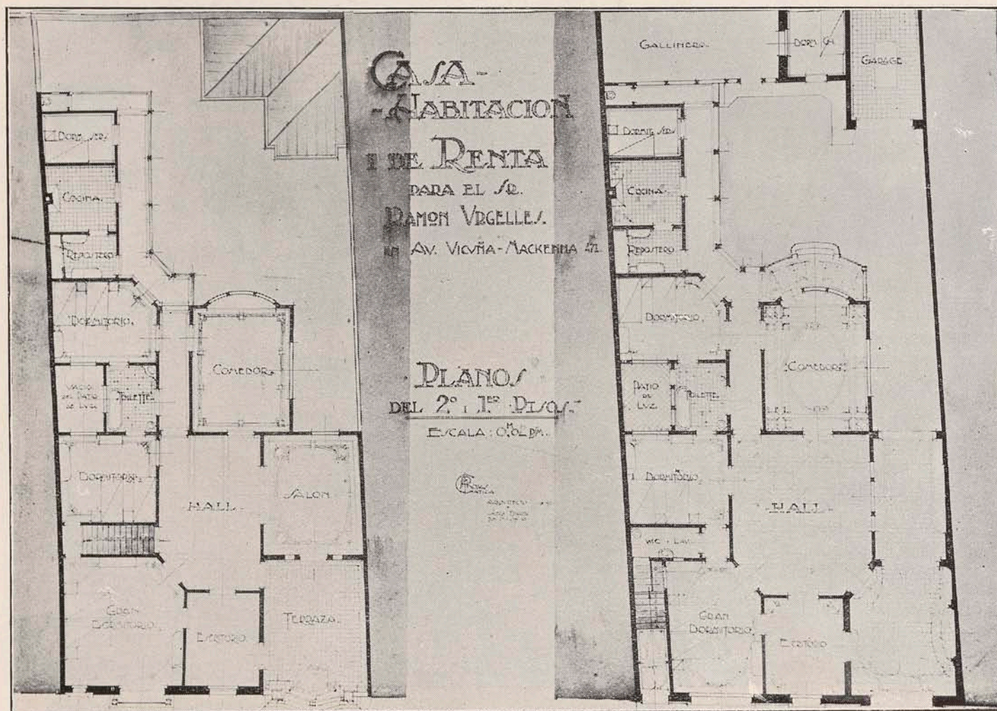
Planos del 1o. y 2o. piso de la propiedad de don Ramón Urgelles, Vicuña Mackenna 47
