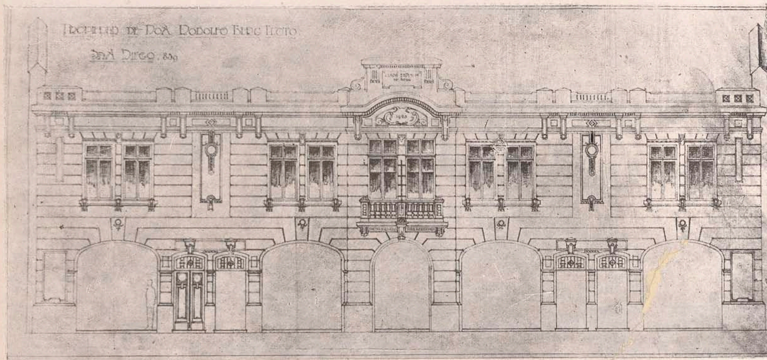
Fachada
