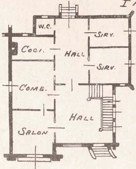
PRIMER PISO
