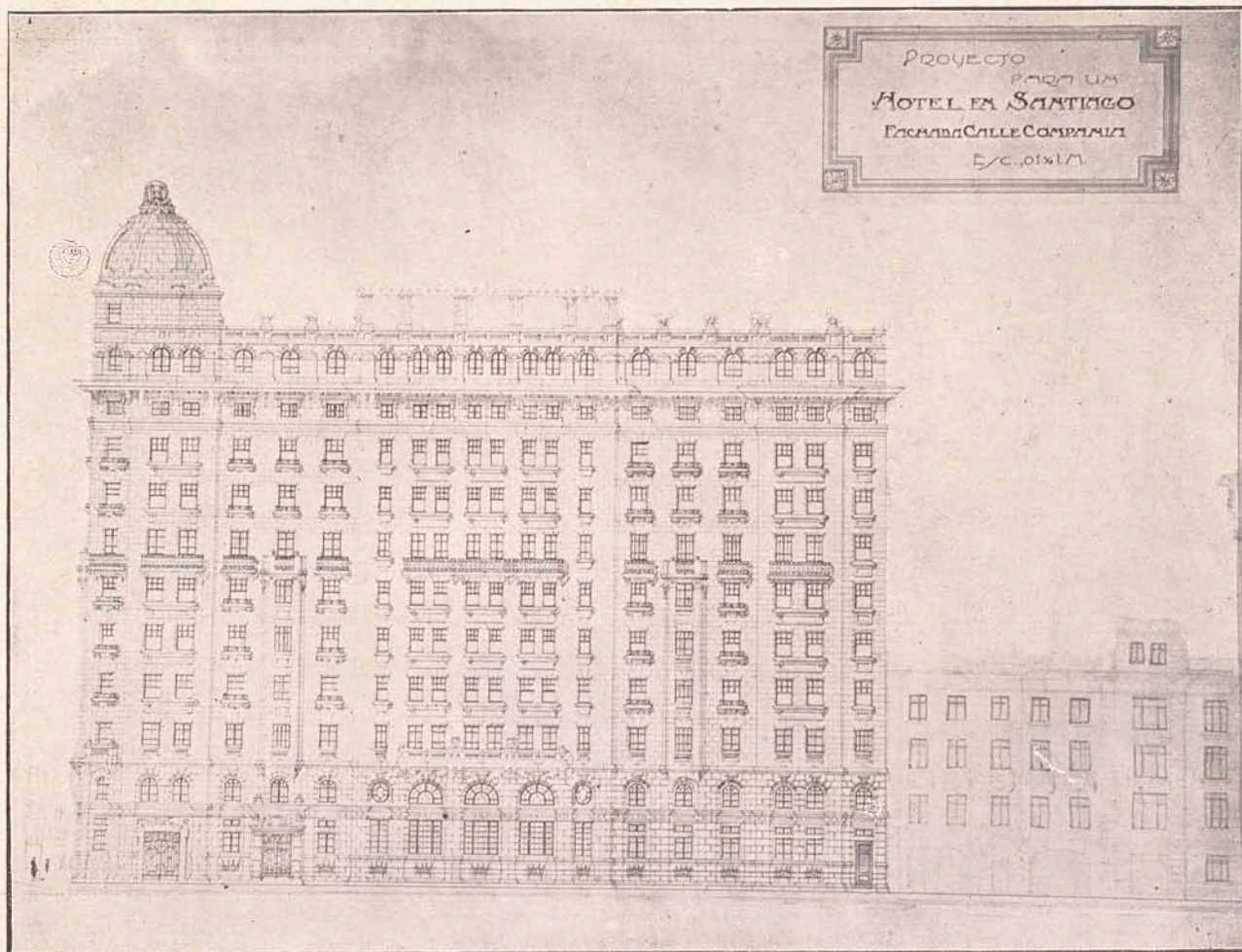
Proyecto final. Fachada calle Compañía
