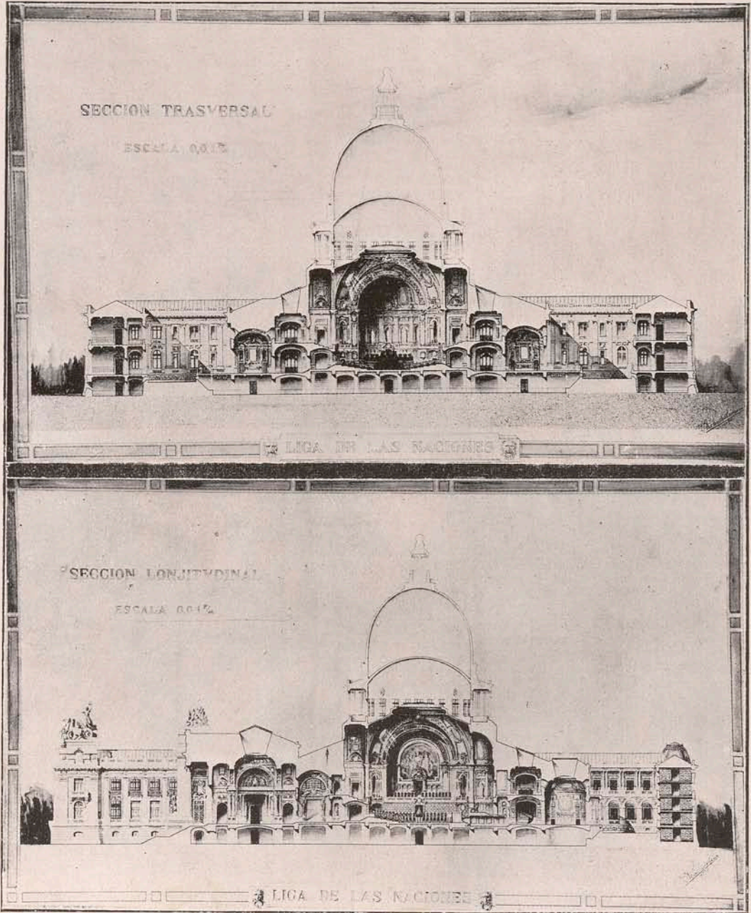
Dos secciones del proyecto final «Liga de las Naciones»
