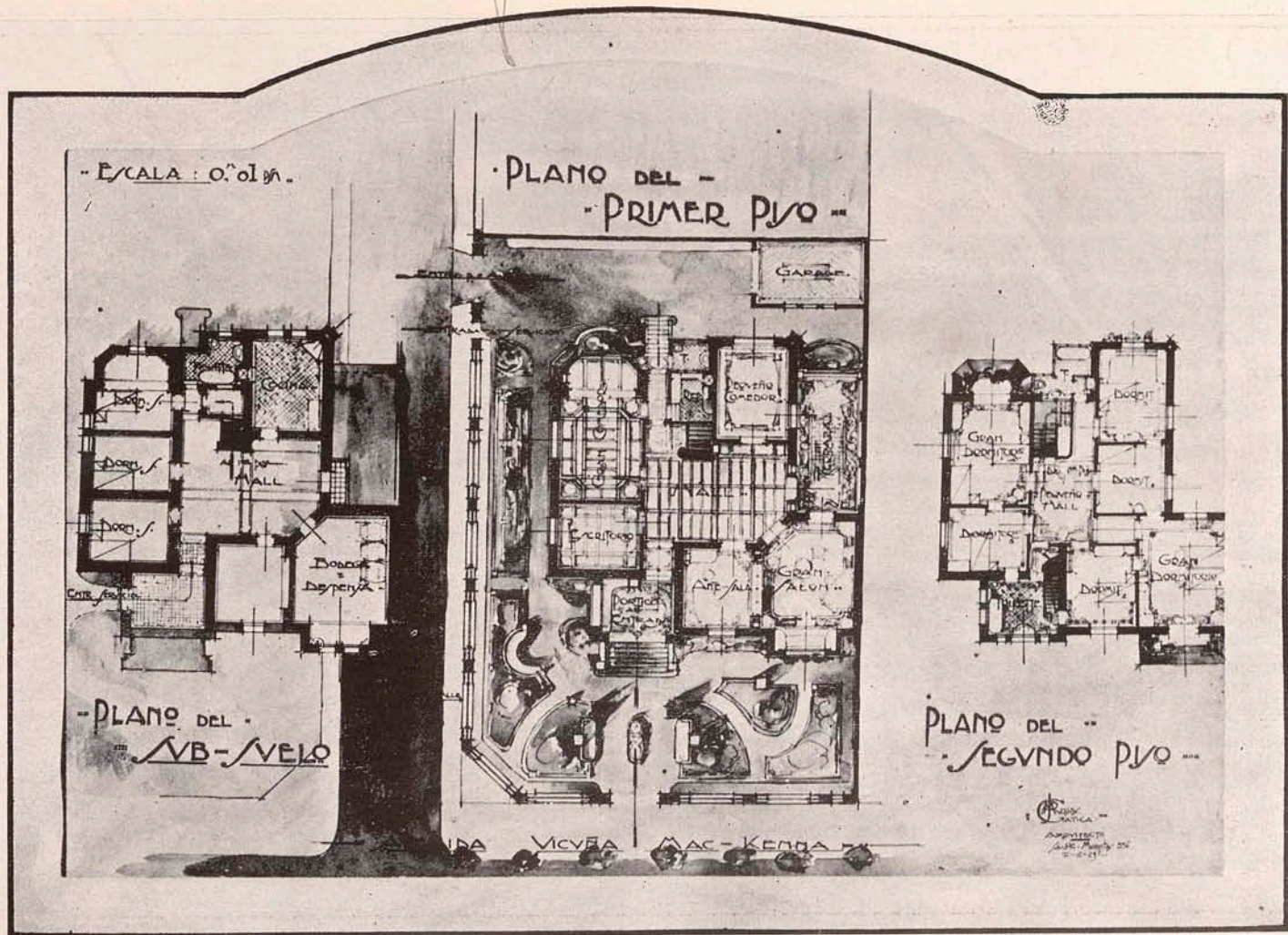
Planos del Chalet en construcción en calle Vicuña Mackenna No. 80.
