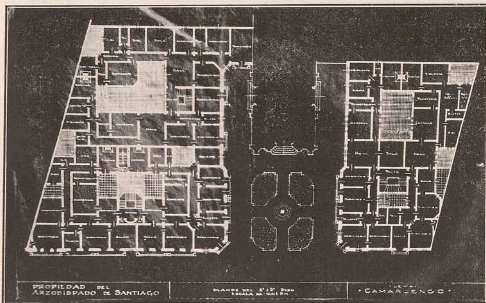
Planos del proyecto
