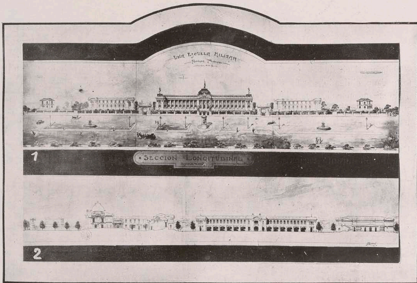
Proyecto para «Una Escuela Militar», con el cual recibió su título. 1 Fachada Principal. 2 Sección Longitudinal.
