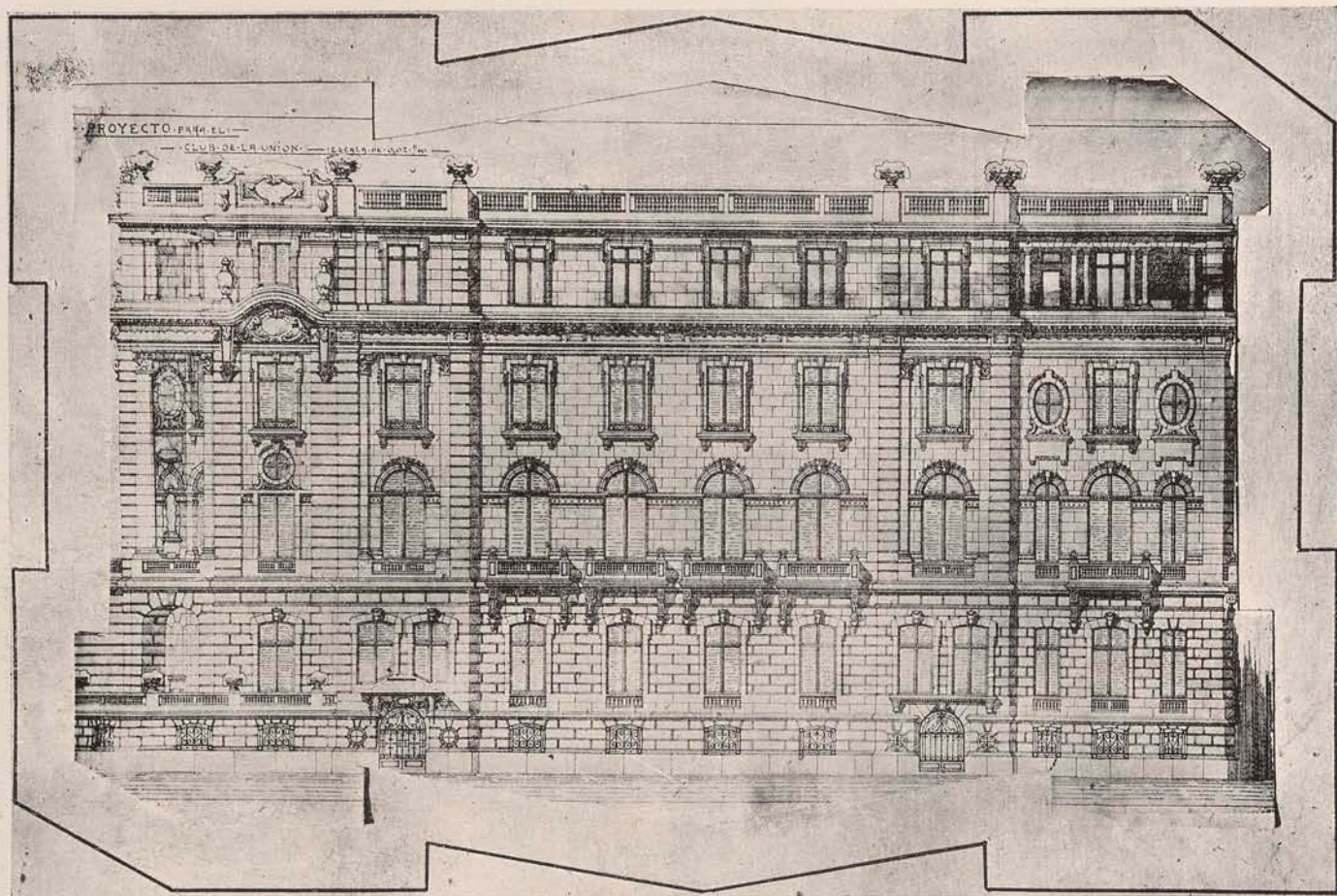
Proyecto del «Club de la Unión» fachada por la calle New York.
