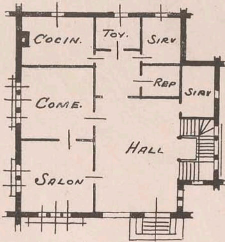
PRIMER PISO
