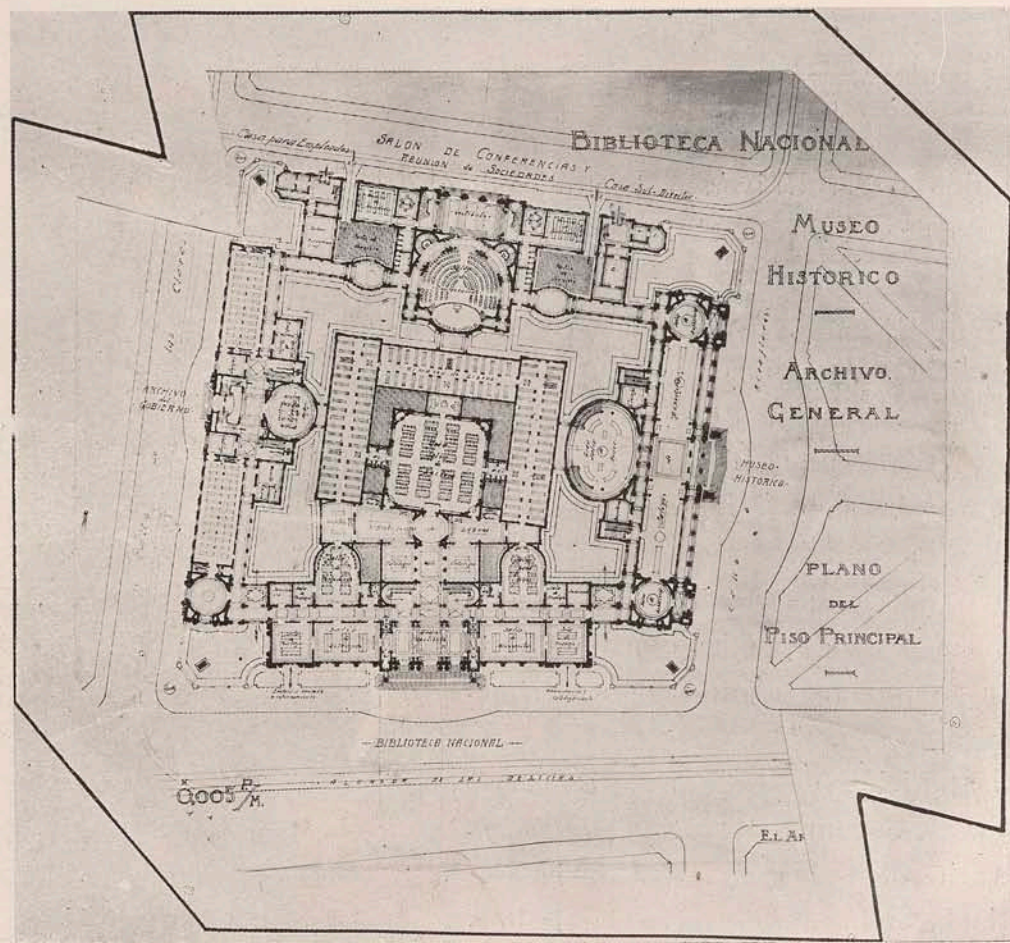
Biblioteca Nacional.—Plano del Piso Principal
