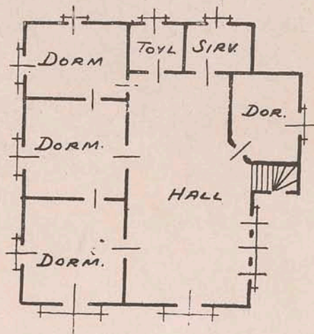
SEGUNDO PISO
