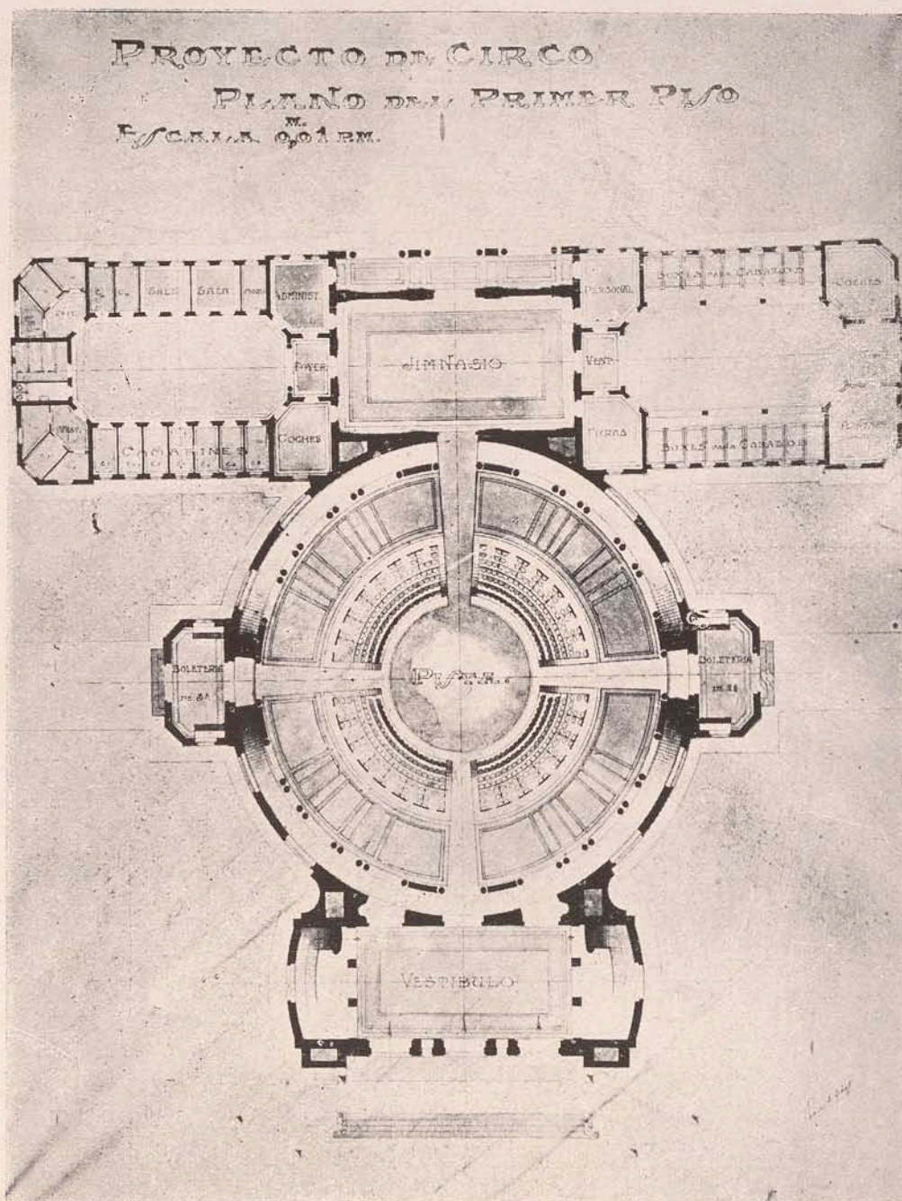
Planta
