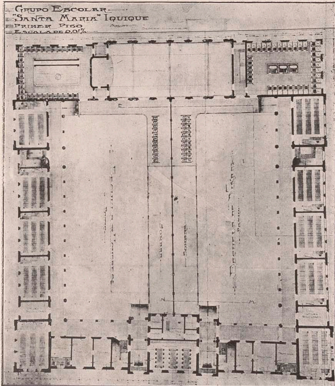
Grupo Escolar de Iquique.—Plantas del primer piso.
