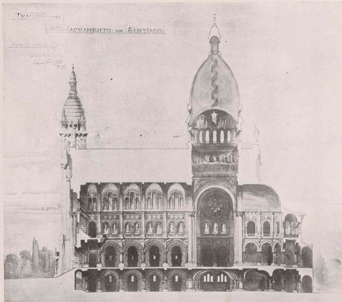
Templo del Santísimo Sacramento. Sección longitudinal
