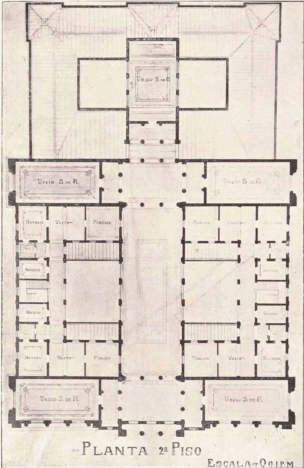
Planta del 2.º Piso del proyecto Final.
