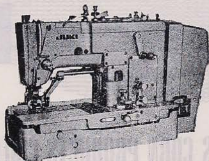
MAQUINA DE HACER OJALES de Doble Pespunte, Alta Velocidad.
