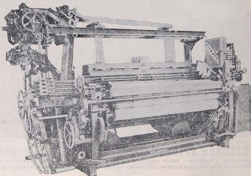
Telar "President" 4C" 148 cm. de ancho útil en el peine, equipado con ratier para dibujo en papel-cartón.
