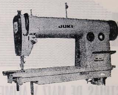
MAQUINA COSTURA RECTA, lubricación automática, 5.500 R.P.M.
